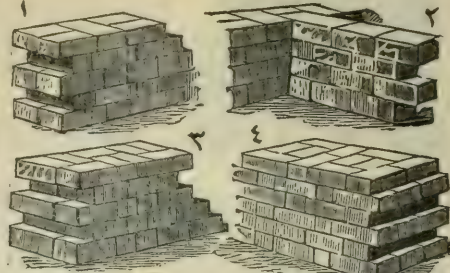
( دیوار )
